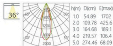
Medium 36°
