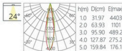
Narrow 24°
