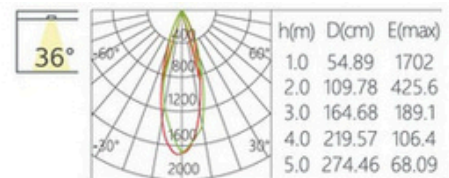
Medium 36°
